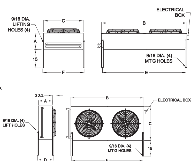
DRAWING - 2 FAN
