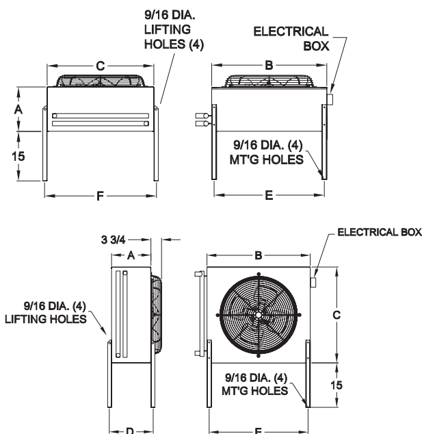
DRAWING - 1 FAN
