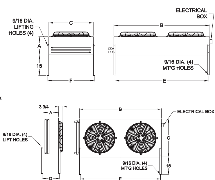
DRAWING - 2 FAN
