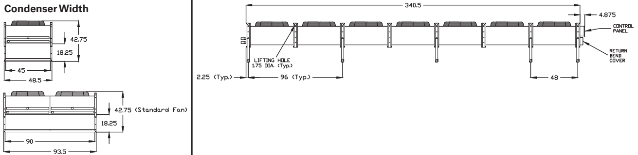
Condenser Width
