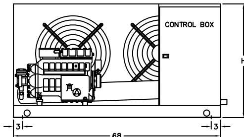
FRONT VIEW - 2 FAN MODEL DE
