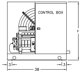
FRONT VIEW - 1 FAN MODEL DE
