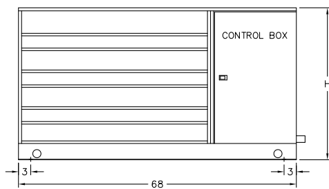
FRONT VIEW - 2 FAN
